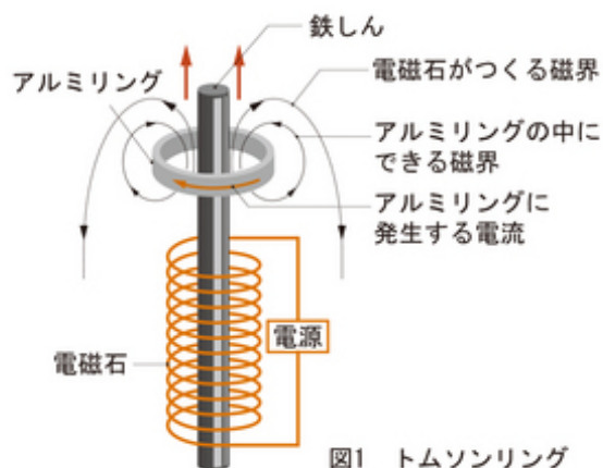
図1 トムソンリング
