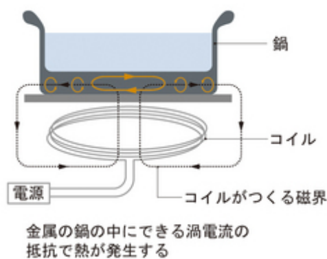
図2 電磁調理器(IH)のしくみ
