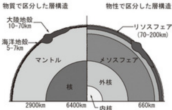
図 地球層構造
